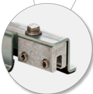
Dettaglio del morsetto S5
