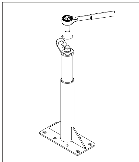
4. Serraggio con chiave dinamometrica (80 Nm)
