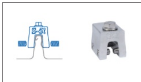
Lamiera RibRoof 465
